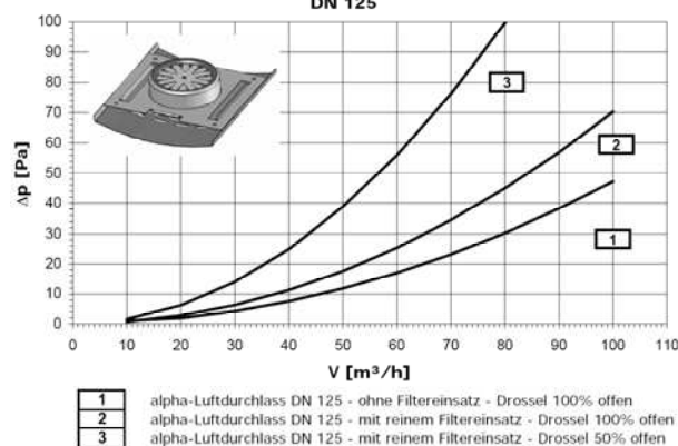
alpha-Luftdurchlass DN 125
