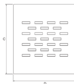
alpha-Luftdurchlass DN 125
